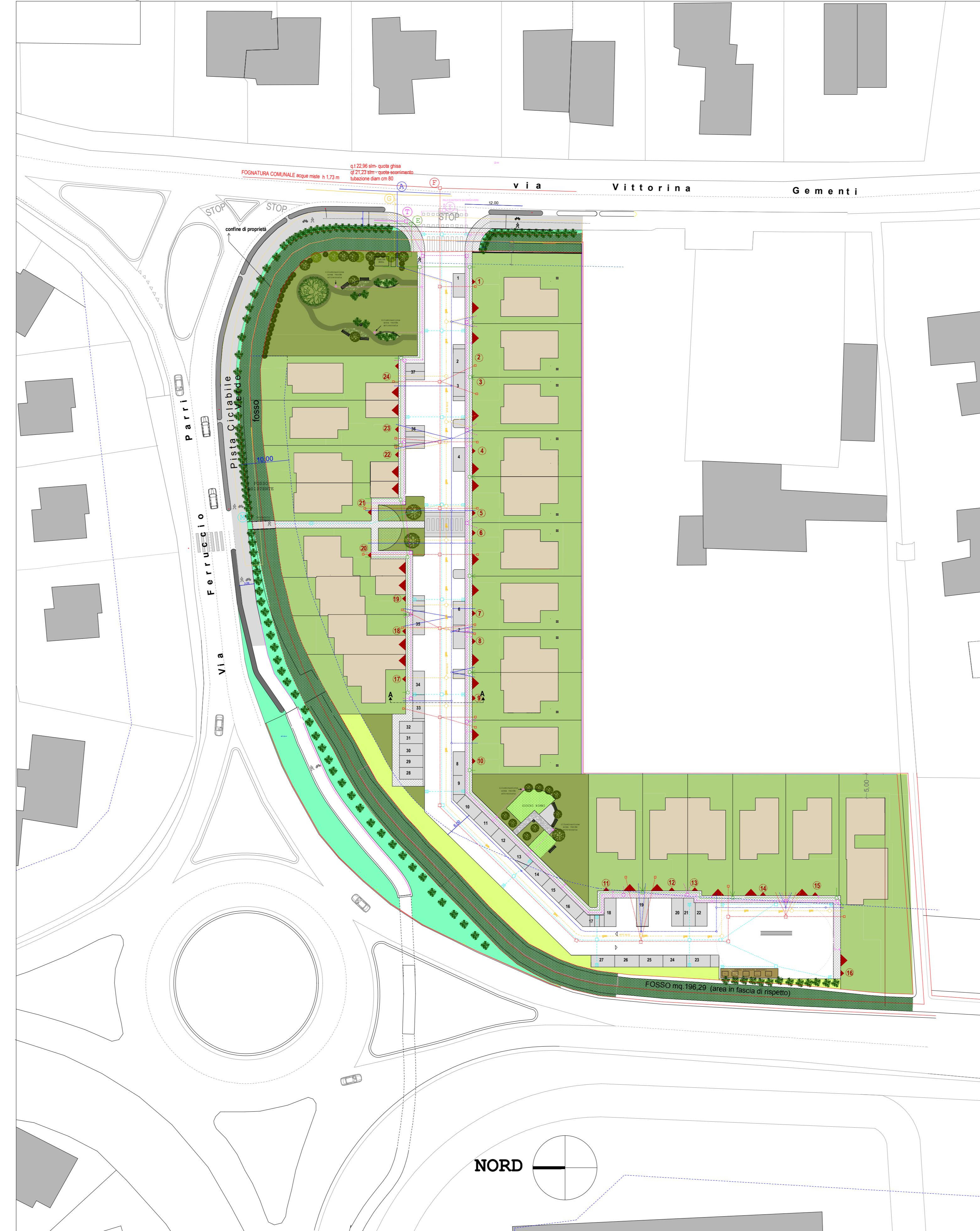
Planimetria generale scala 1:500
