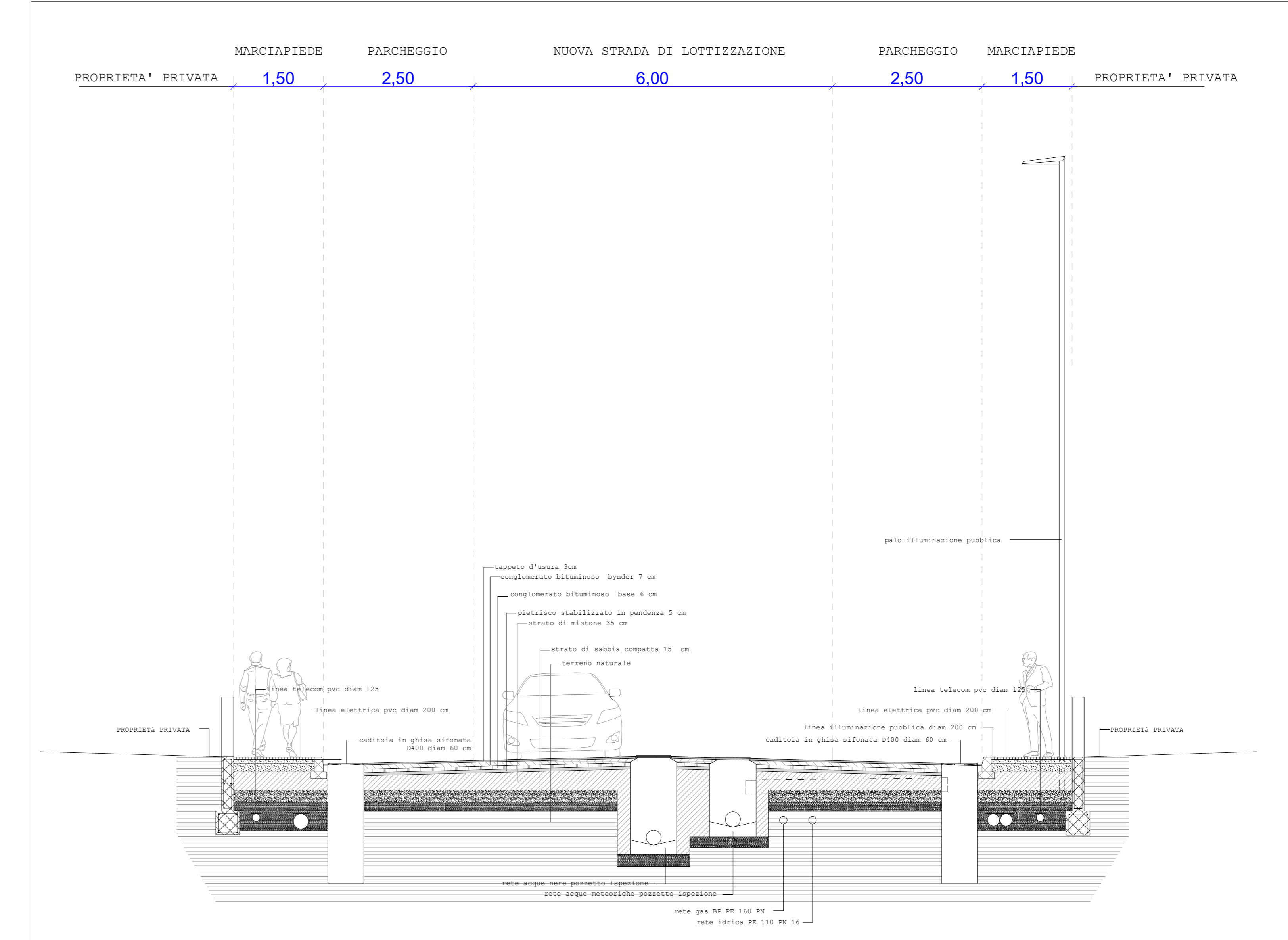
Sezione nuova strada di lottizzazione AA - scala 1:50
