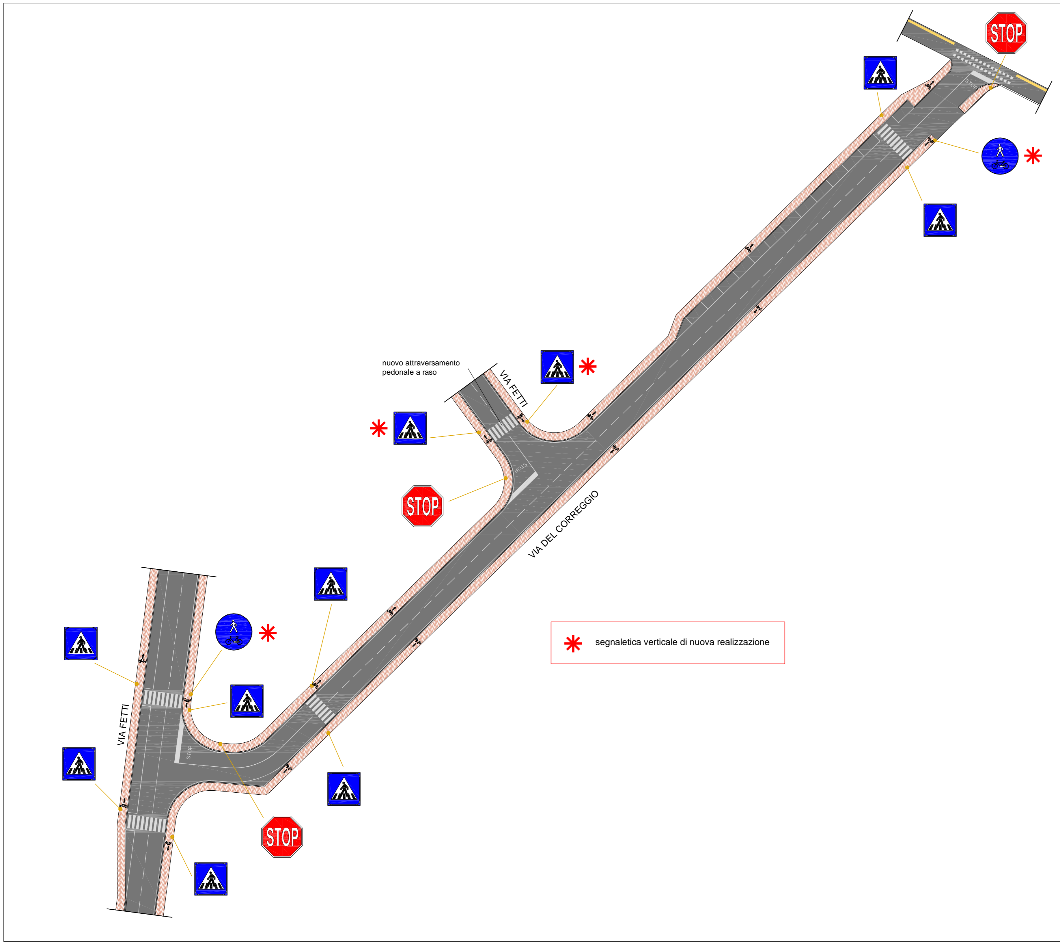
VIA DEL CORREGGIO - SEGNALETICA STRADALE scala 1:500
